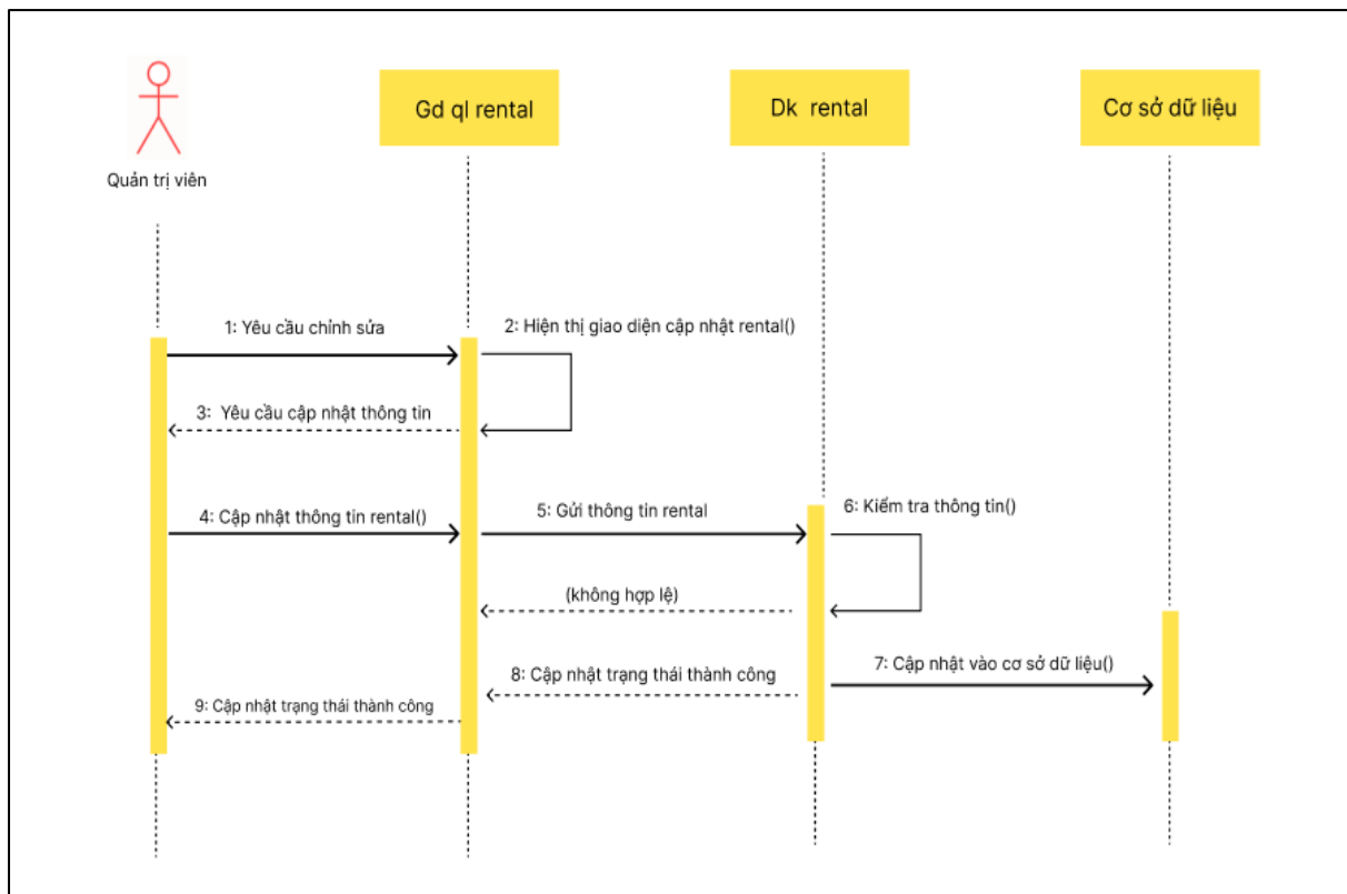
Hình 2.12. Biểu đồ tuần tự chức năng cập nhật trạng thái đặt xe
