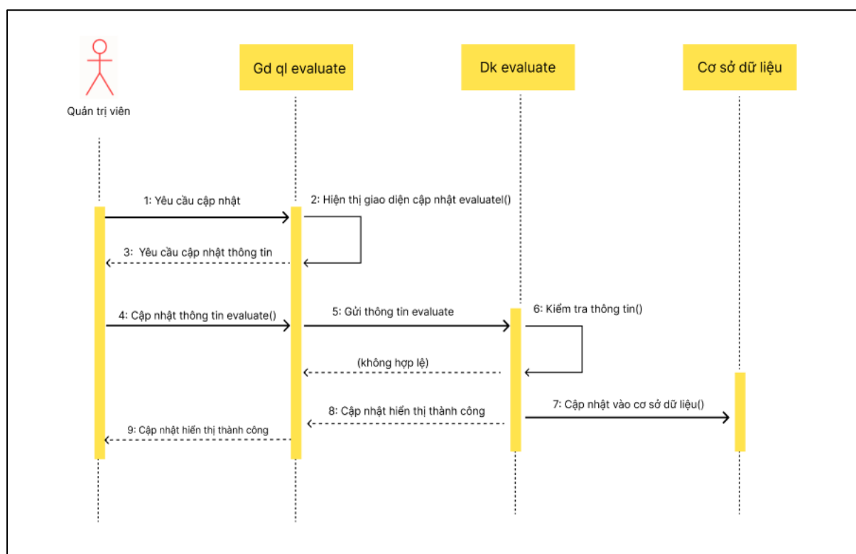
Hình 2.14. Biểu đồ tuần tự chức năng thêm/sửa/xóa đánh giá
