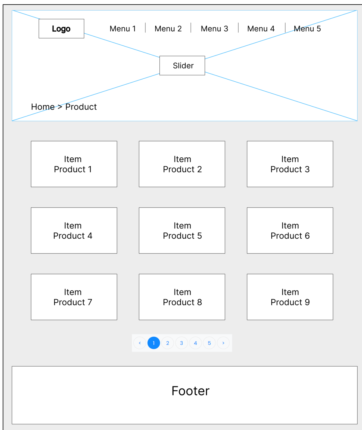
Hình 2.19. Mô hình tổng thể giao diện sản phẩm
