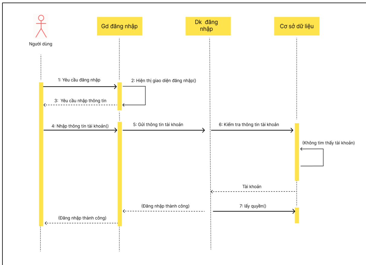
Hình 2.7. Biểu đồ tuần tự chức năng đăng nhập tài khoản quản trị viên
