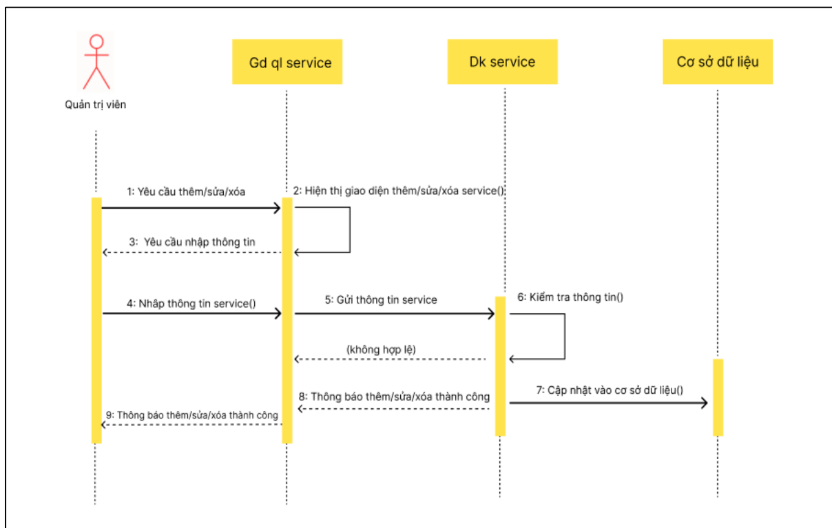
Hình 2.13. Biểu đồ tuần tự chức năng thêm/sửa/xóa dịch vụ
