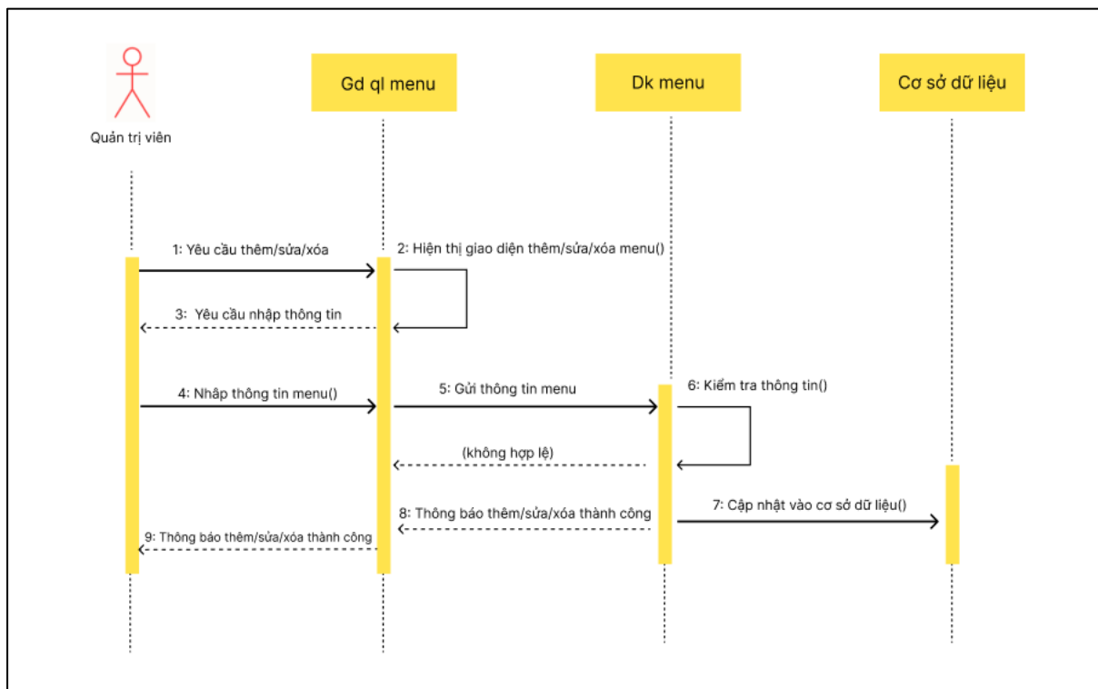
Hình 2.8. Biểu đồ tuần tự chức năng thêm/sửa/xóa thanh thực đơn
