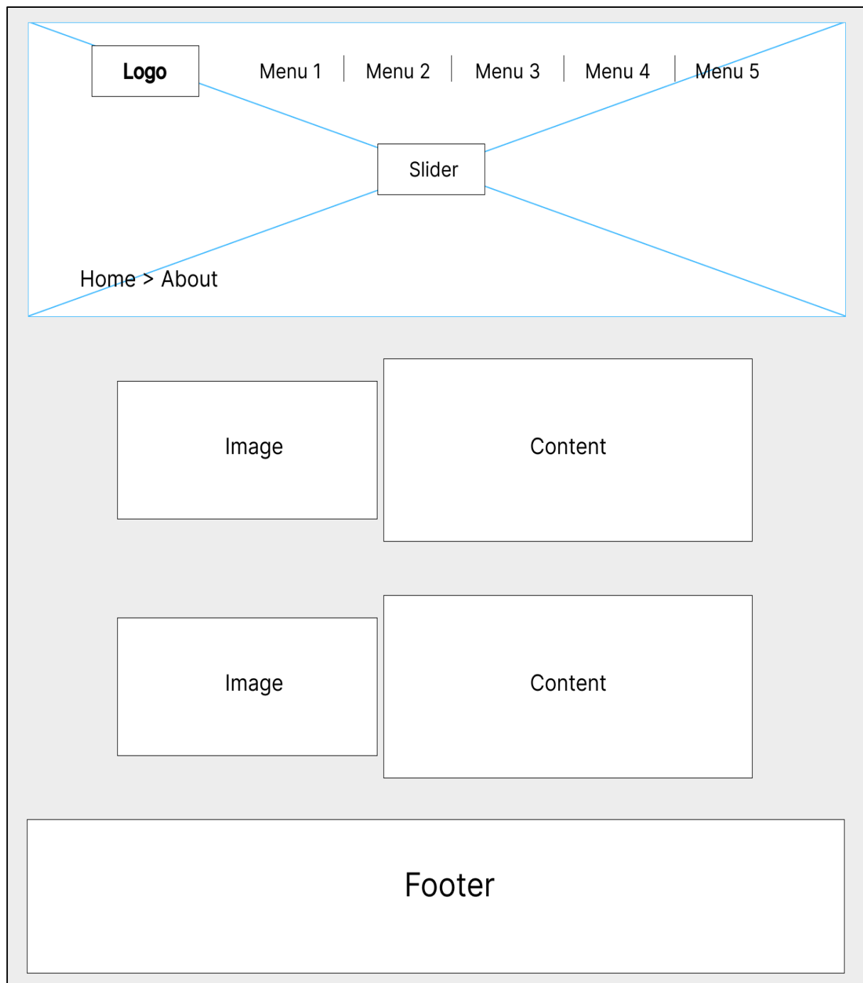
Hình 2.18. Mô hình tổng thể giao diện giới thiệu
