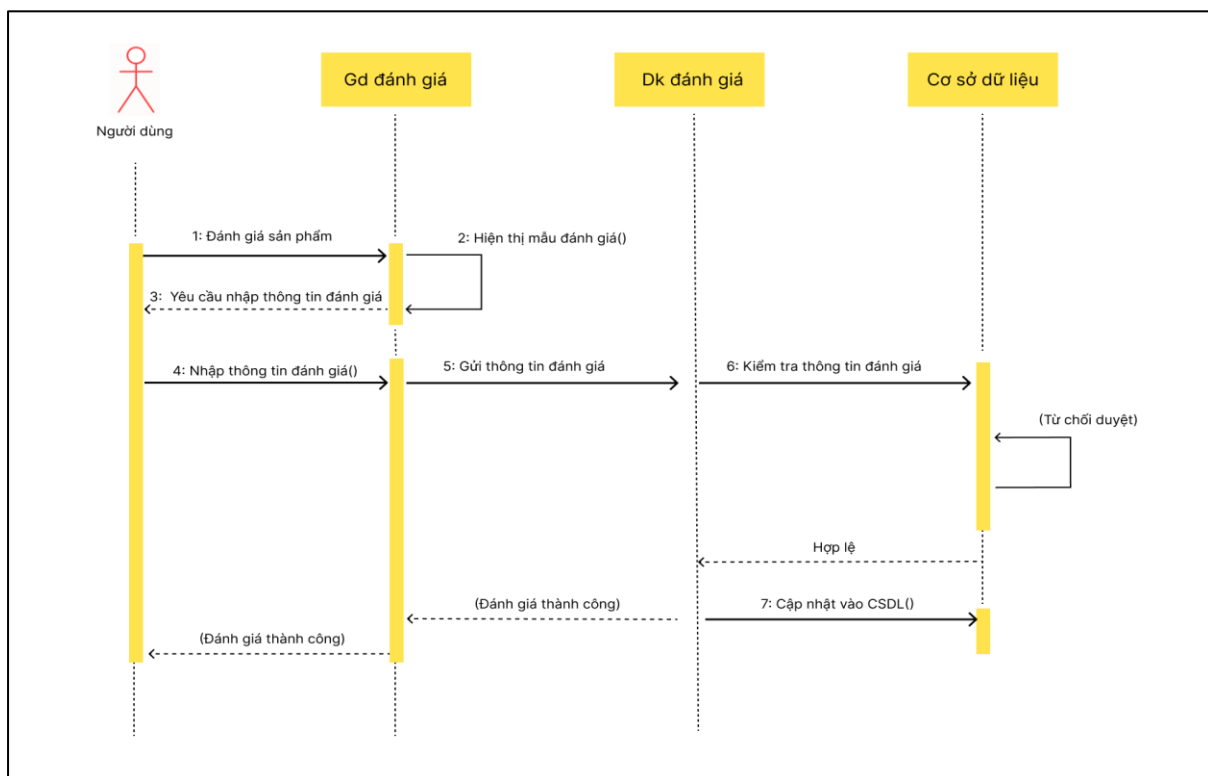
Hình 2.5. Biểu đồ tuần tự chức năng đánh giá sản phẩm
