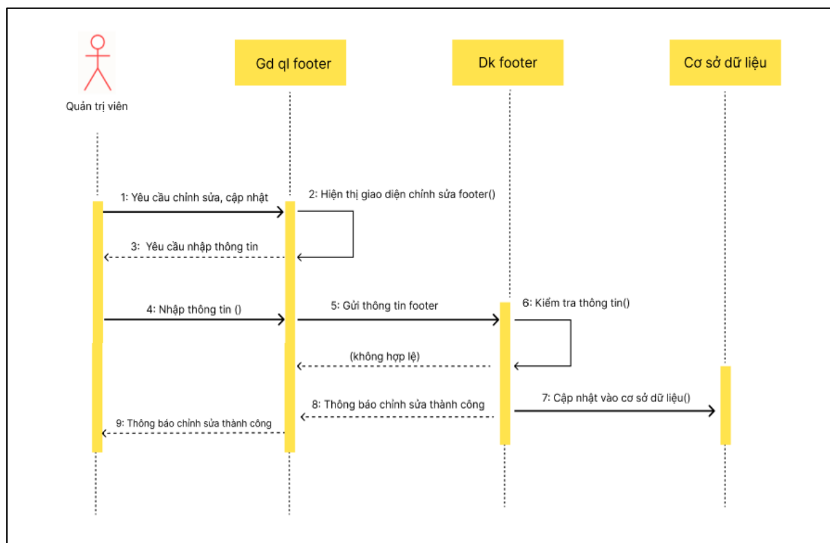
Hình 2.15. Biểu đồ tuần tự chức năng chỉnh sửa, cập nhật footer
