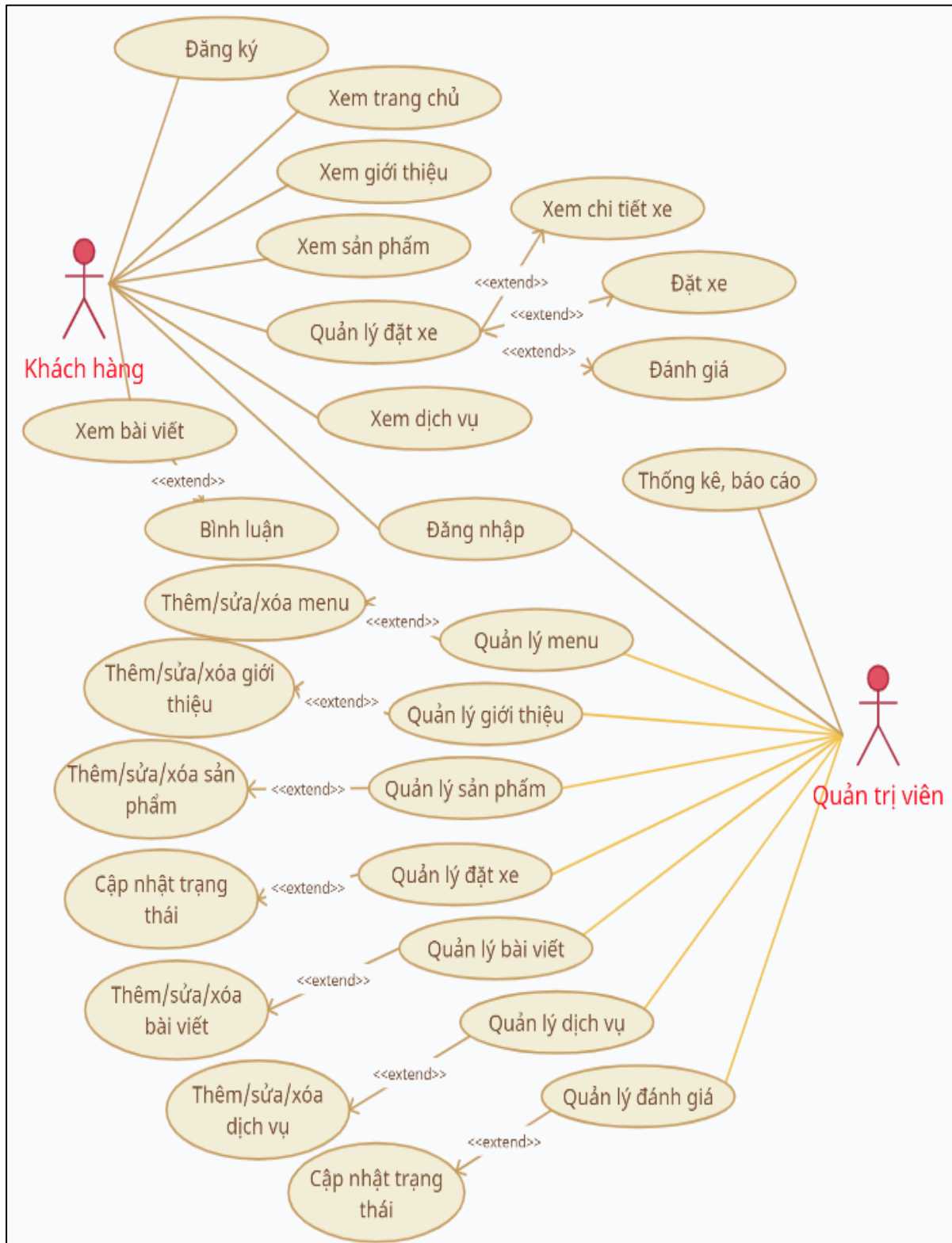
Hình 2.1. Biểu đồ ca sử dụng của hệ thống
