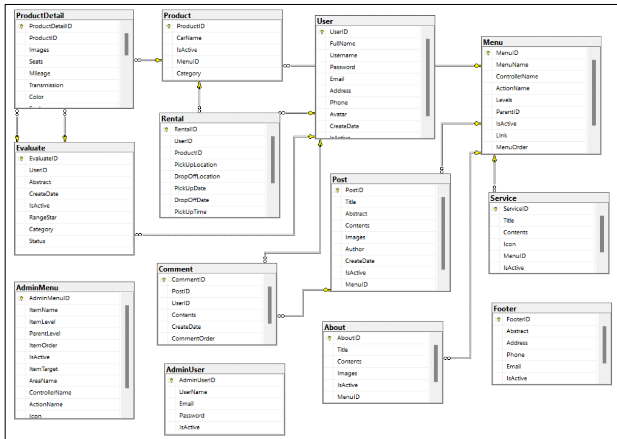
Hình 2.16. Biểu đồ phân lớp của hệ thống
