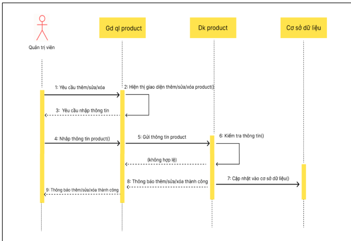
Hình 2.10. Biểu đồ tuần tự chức năng thêm/sửa/xóa sản phẩm
