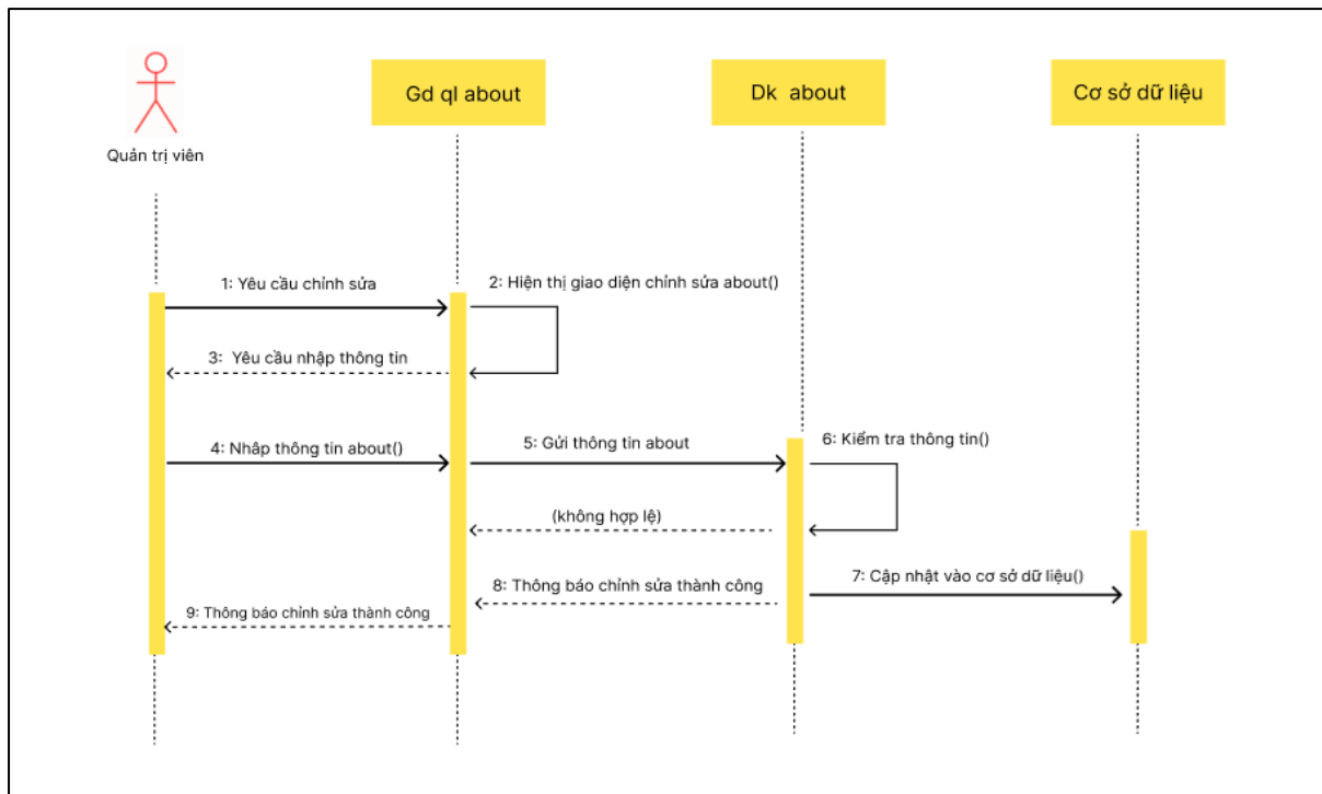
Hình 2.11. Biểu đồ tuần tự chức năng chỉnh sửa giới thiệu
