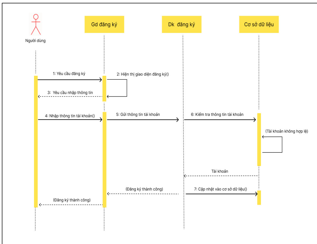
Hình 2.2. Biểu đồ tuần tự chức năng đăng ký tài khoản
