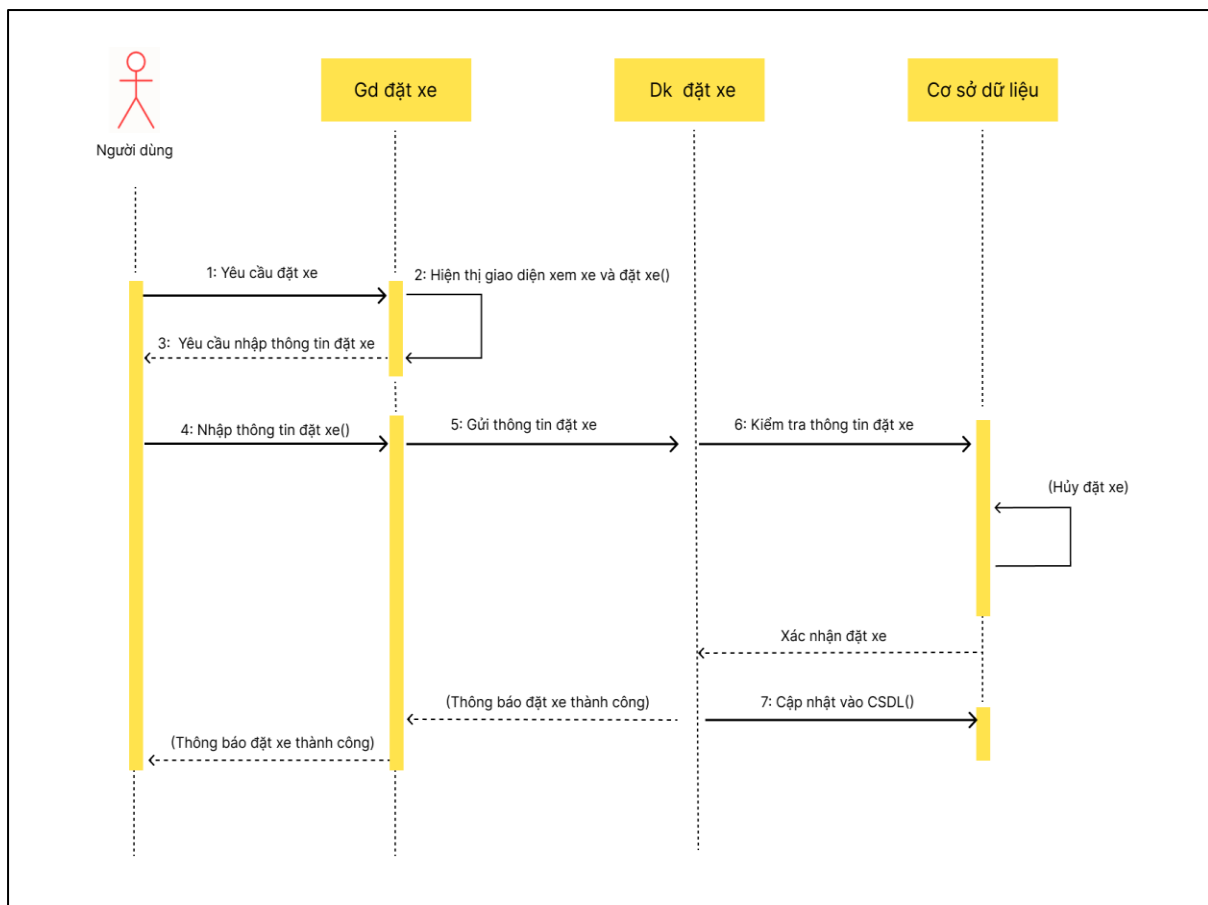
Hình 2.4. Biểu đồ tuần tự chức năng đặt xe
