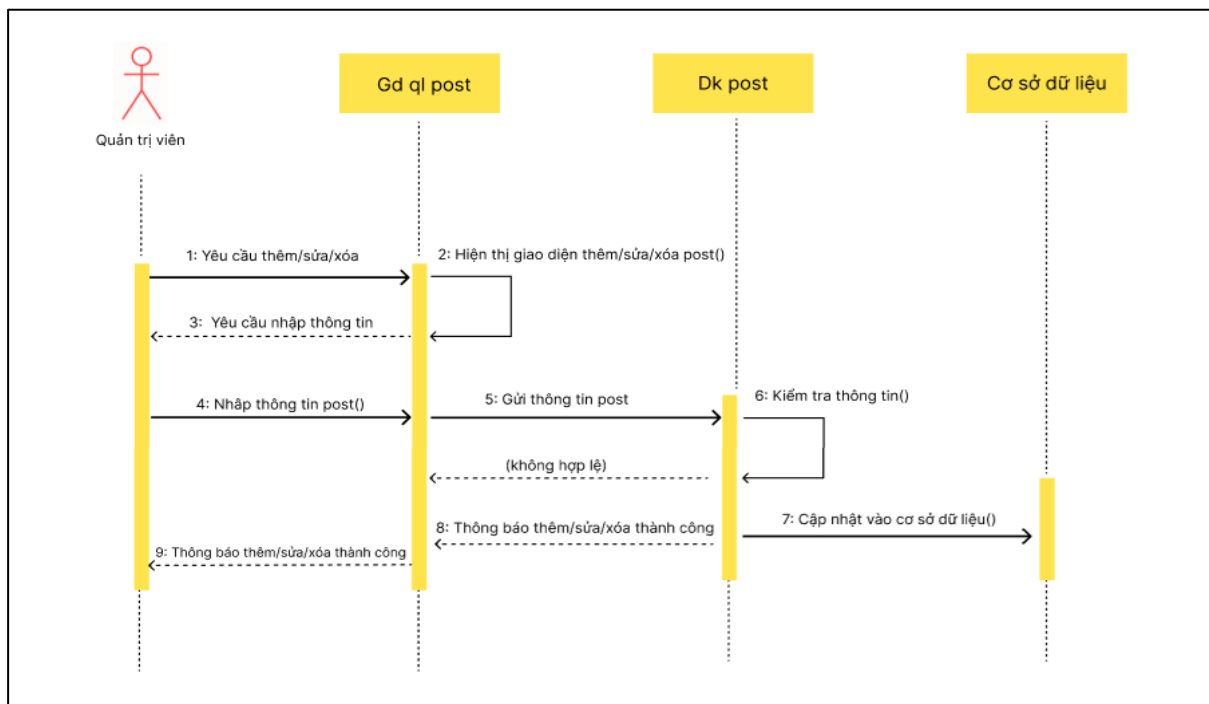
Hình 2.9. Biểu đồ tuần tự chức năng thêm/sửa/xóa bài viết
