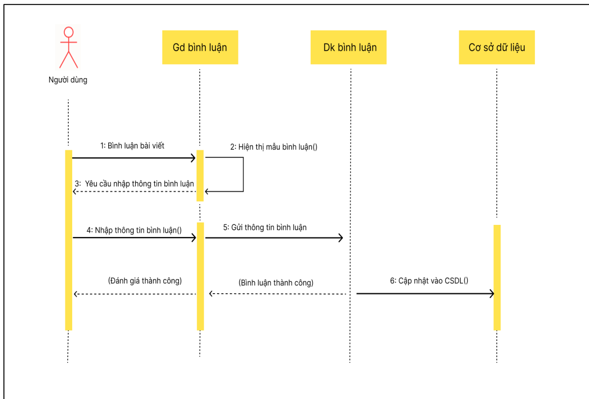
Hình 2.6. Biểu đồ tuần tự chức năng bình luận bài viết
