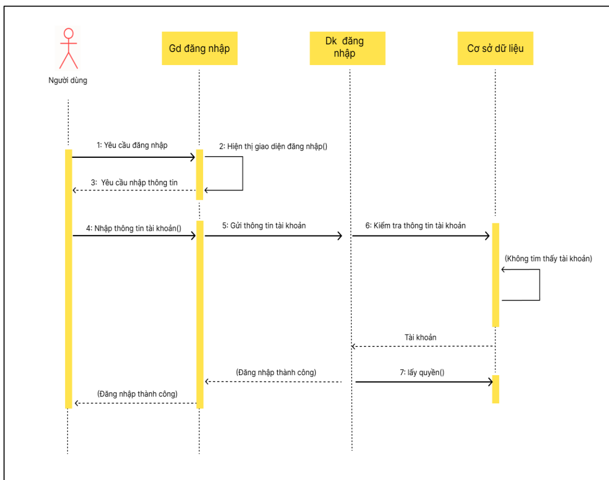
Hình 2.3. Biểu đồ tuần tự chức năng đăng nhập tài khoản người dùng
