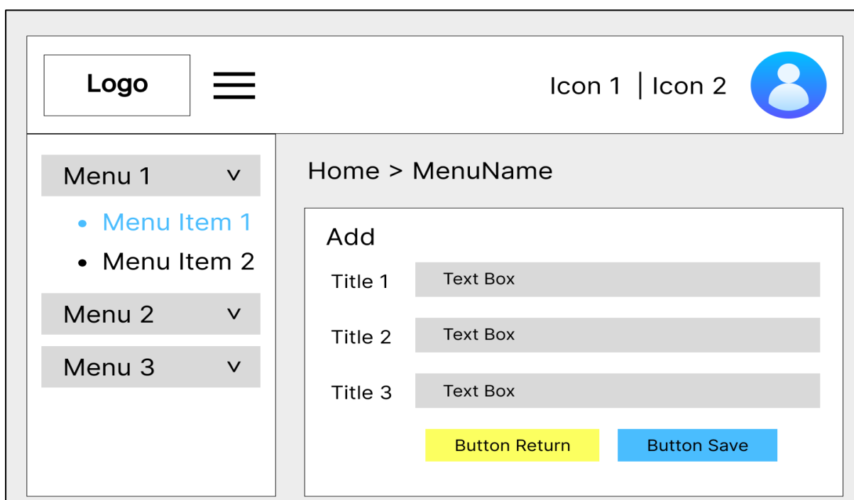
Hình 2.26. Mô hình tổng thể giao diện AdminmenuDetail
